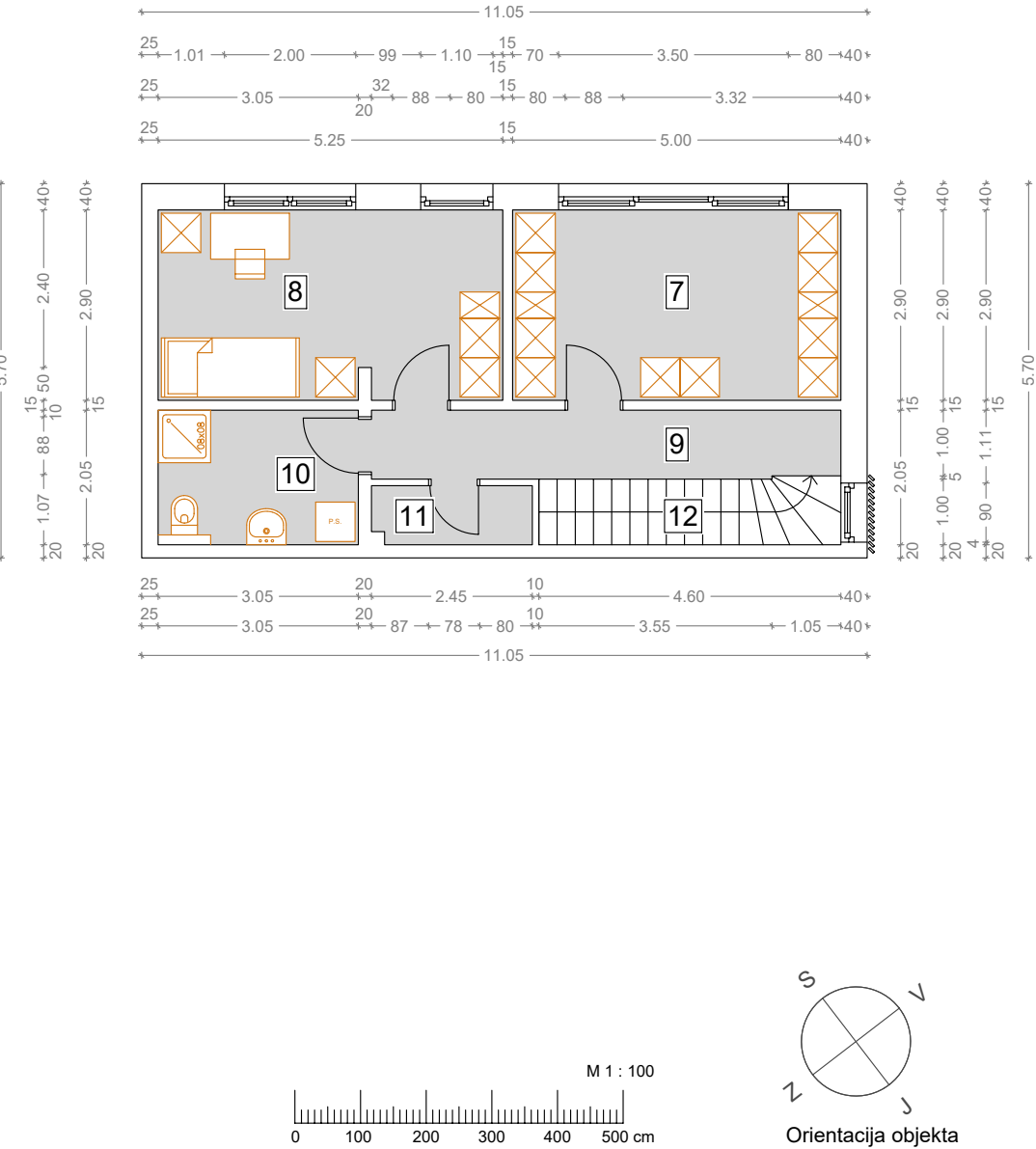
TLORIS NADSTROPJA
