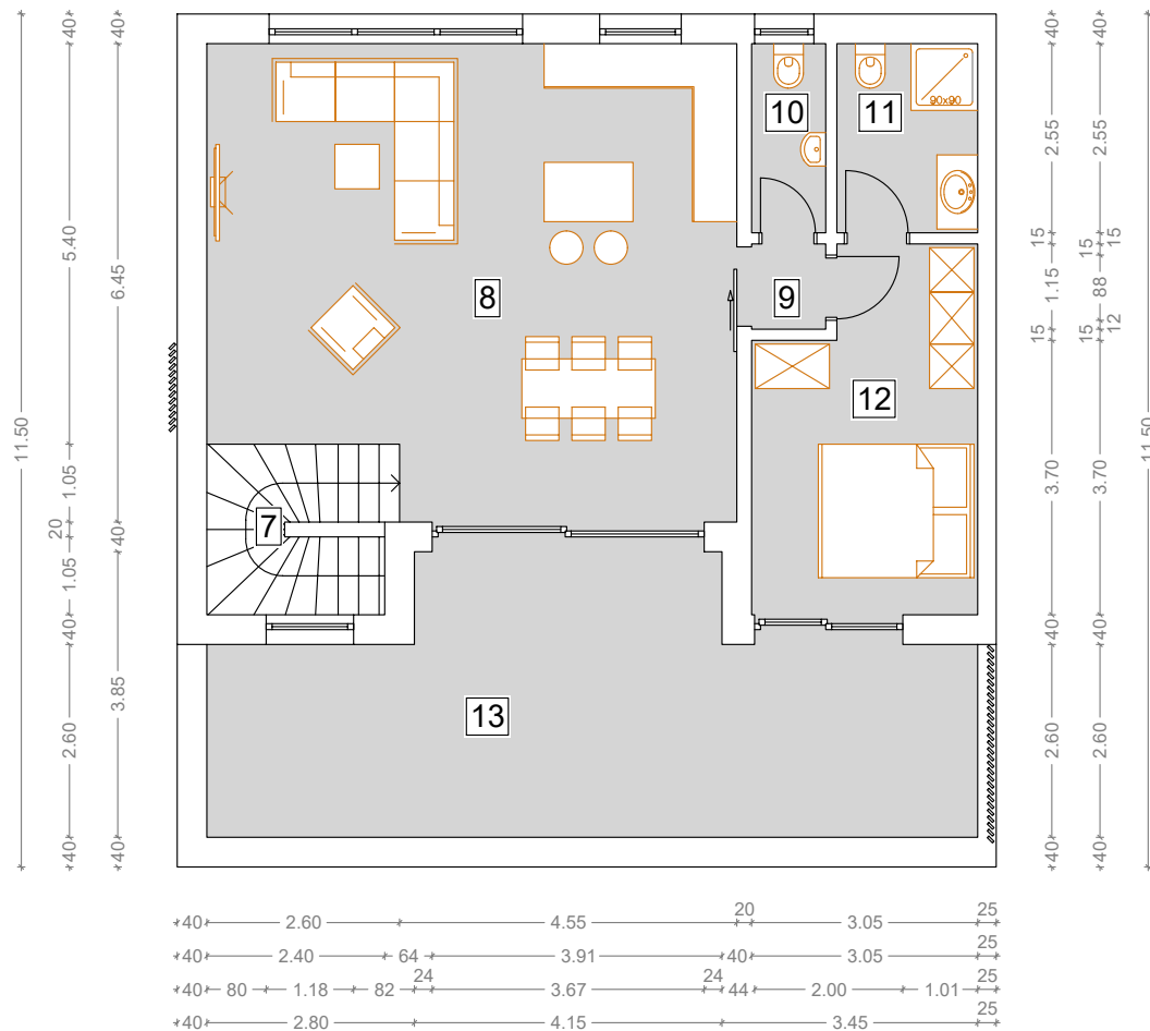
TLORIS 2. NADSTROPJA
