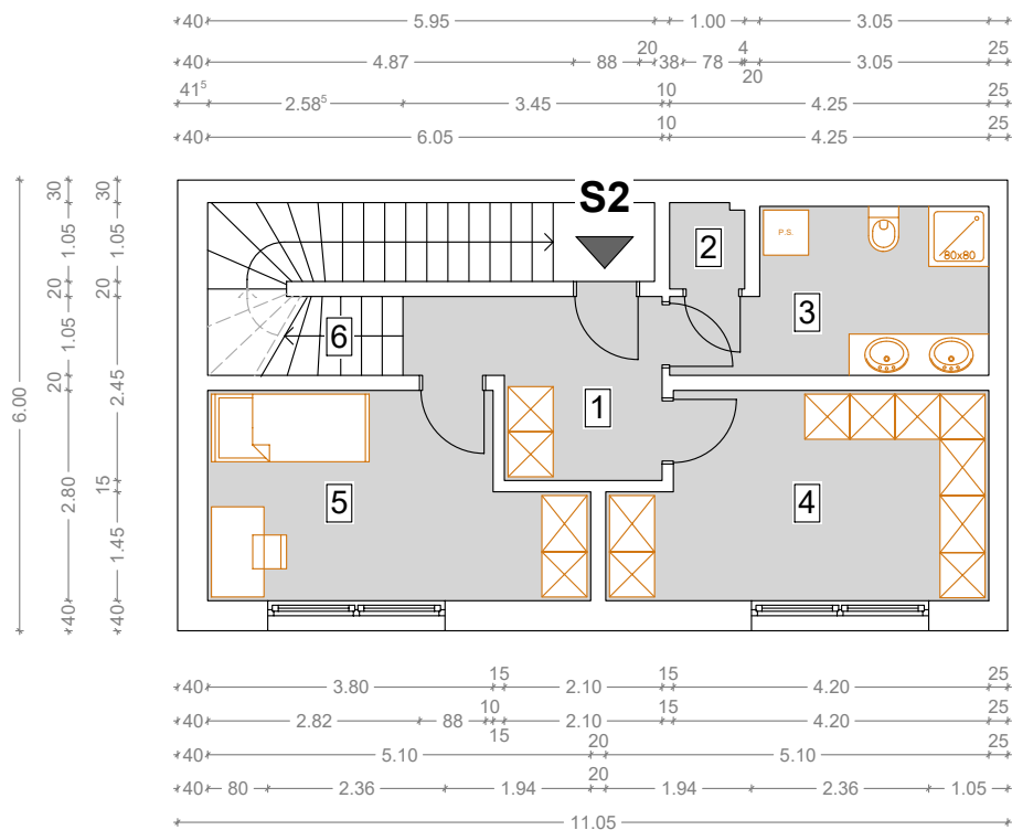
TLORIS 1. NADSTROPJA
